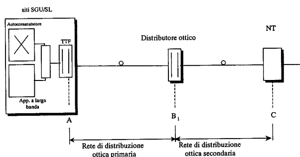
Fig. 1.2. Rete di distribuzione in fibra ottica.
